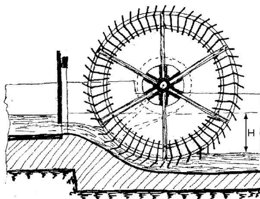
Fig. 33 : Illustration d'une roue dite en dessous. (Schnelle 2012, 82).
