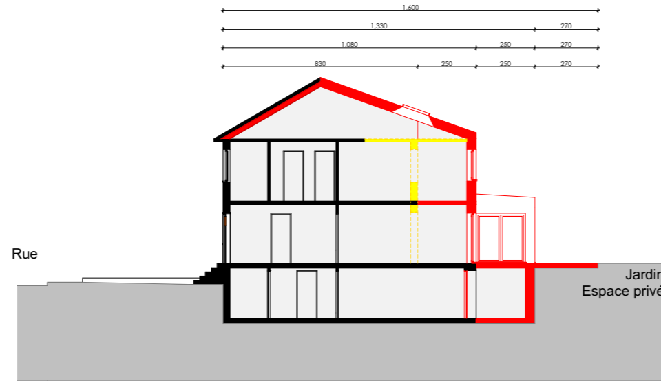
Coupe projetée
