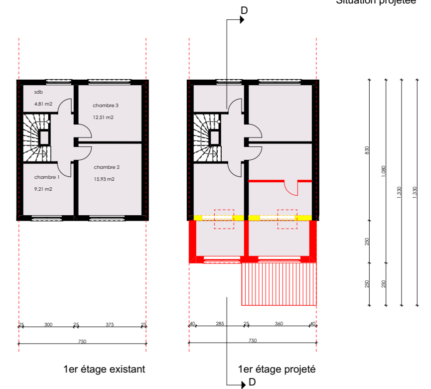
Situation projetée
