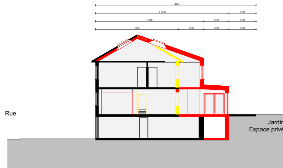
Coupe projetée
