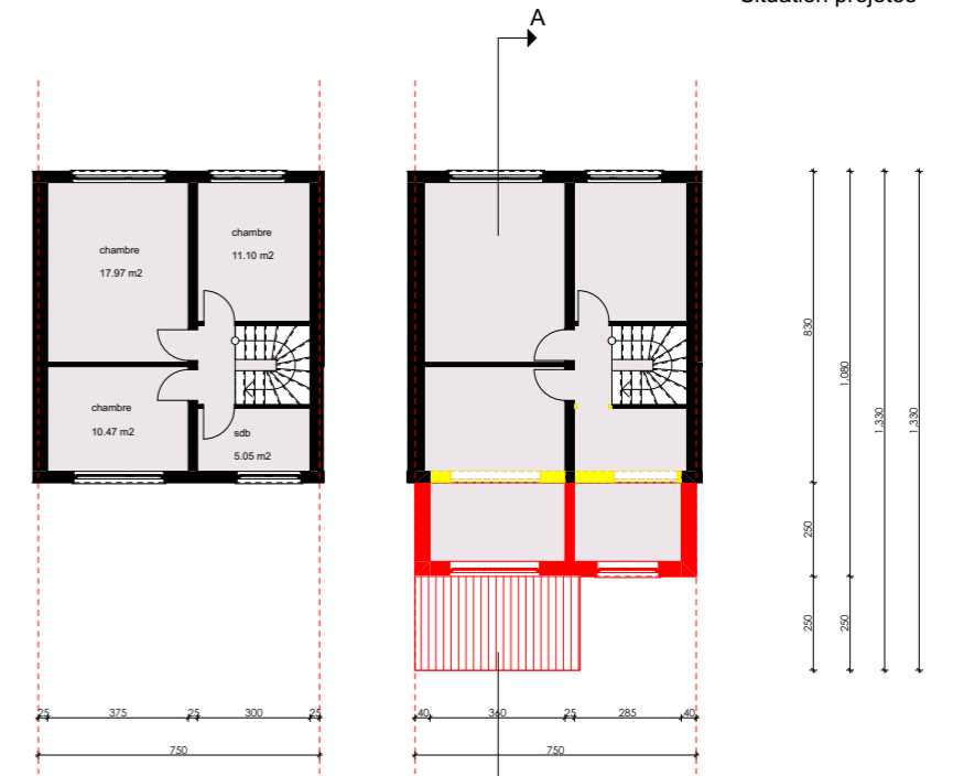
1er étage existant
