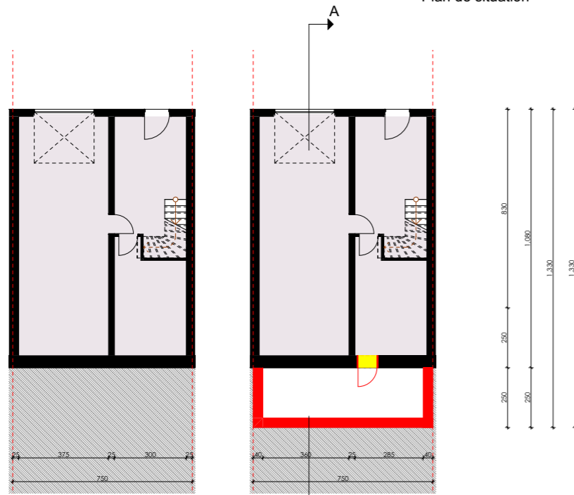
Sous sol existant
