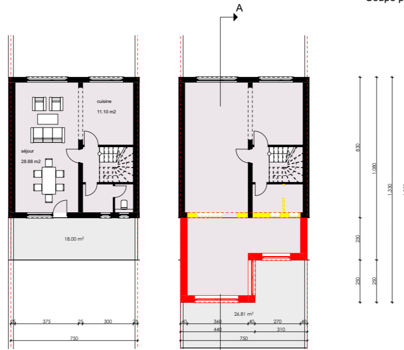
RDC existant
