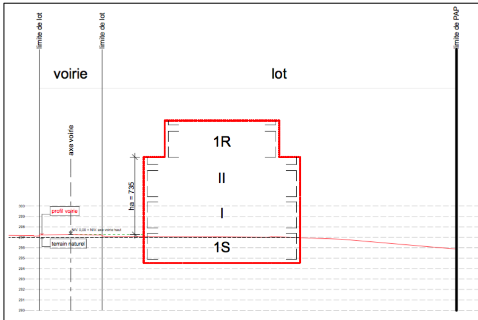
Image 1 : Croquis explicatif pour la définition de la hauteur à l'acrotère
