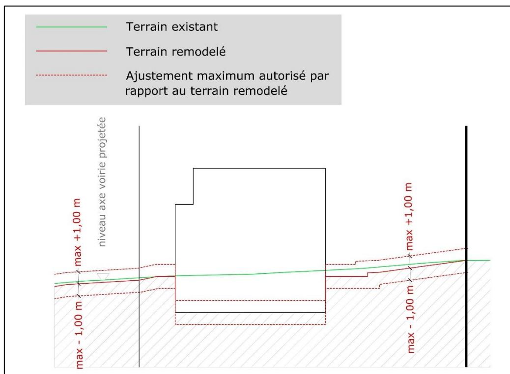
Image 3 : Croquis explicatif pour les ajustements autorisés par rapport au terrain remodelé
