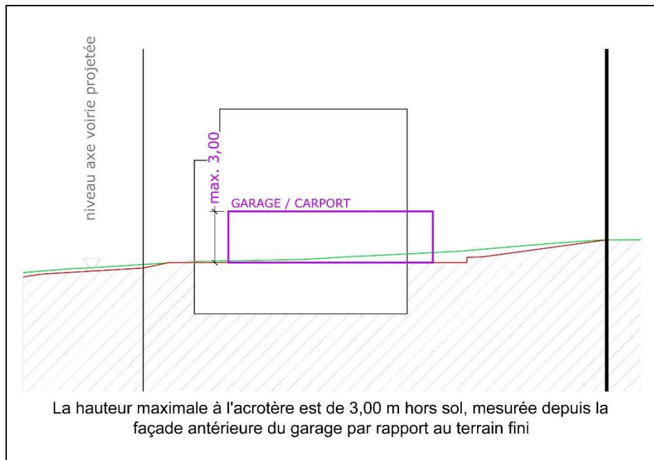
Image 3 : Croquis explicatif pour la définition de la hauteur à l'acrotère des garages/carport
